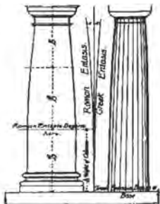
entasis
